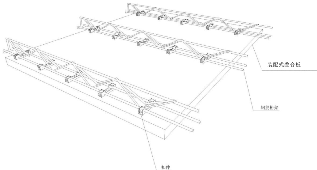
图 4.2.1 钢筋桁架装配式叠合板示意图
